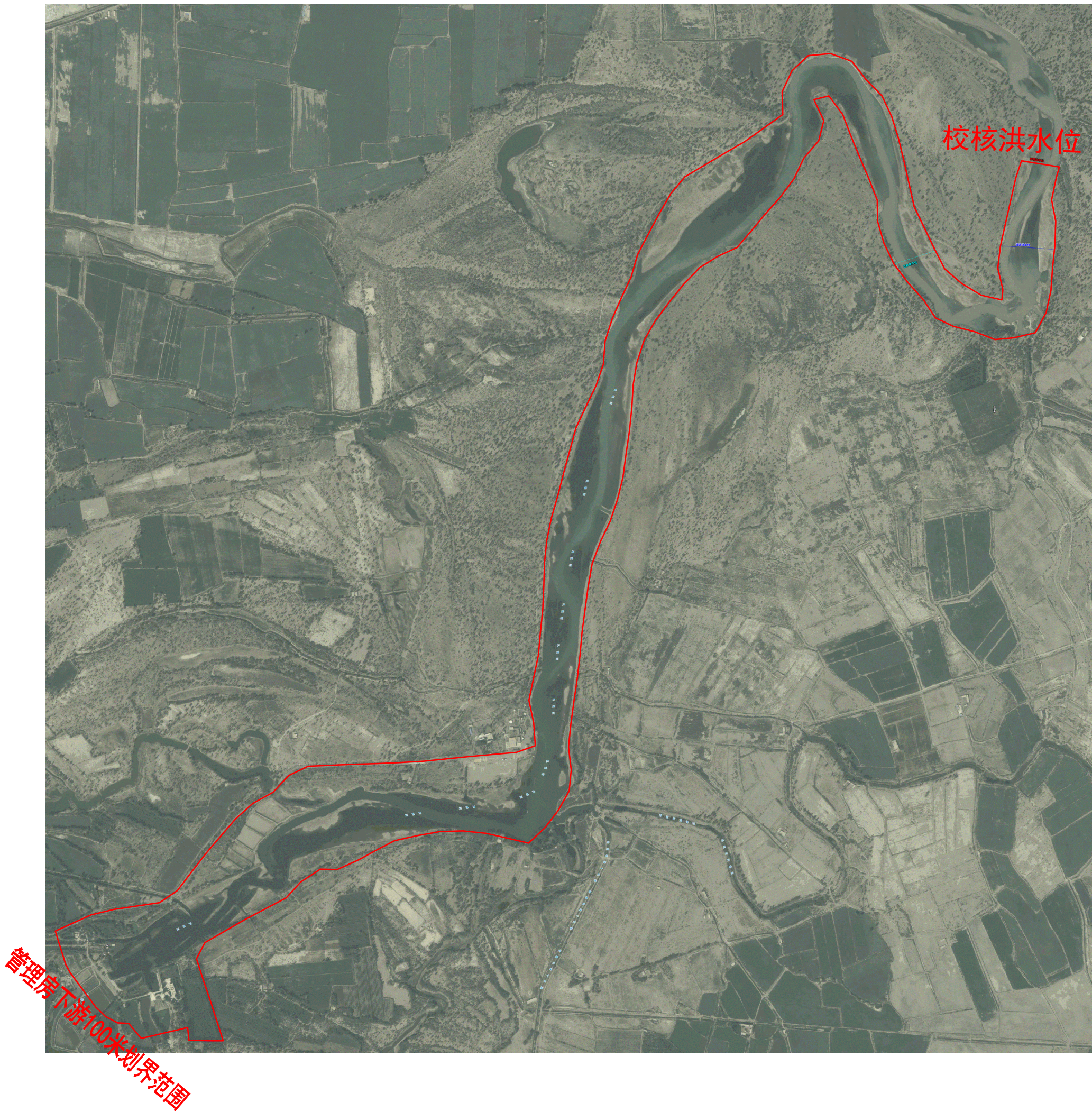
普惠水库校核洪水位及管理房划界图
